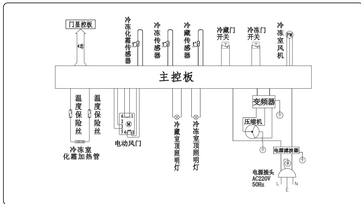
电路图 (BCD-593WD03BZWS/BCD-593WD03GBWG)
