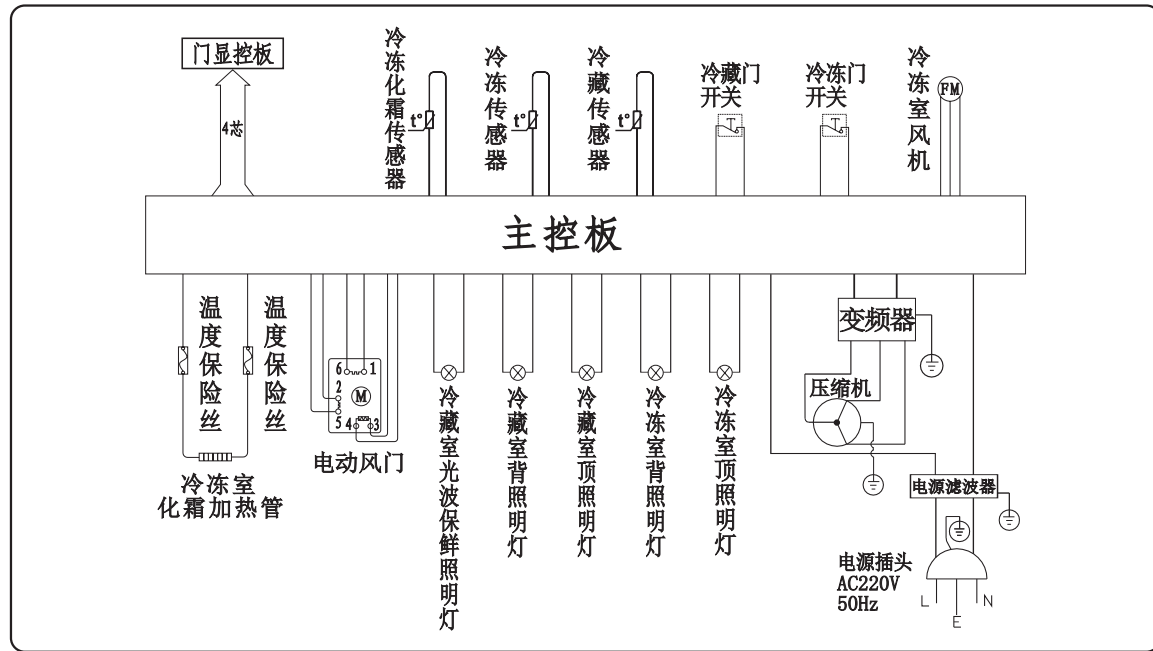
电路图 (BCD-593WDGBW)
