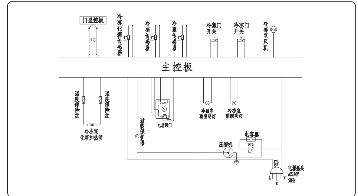
电路图 (BCD-593WDGAW)
