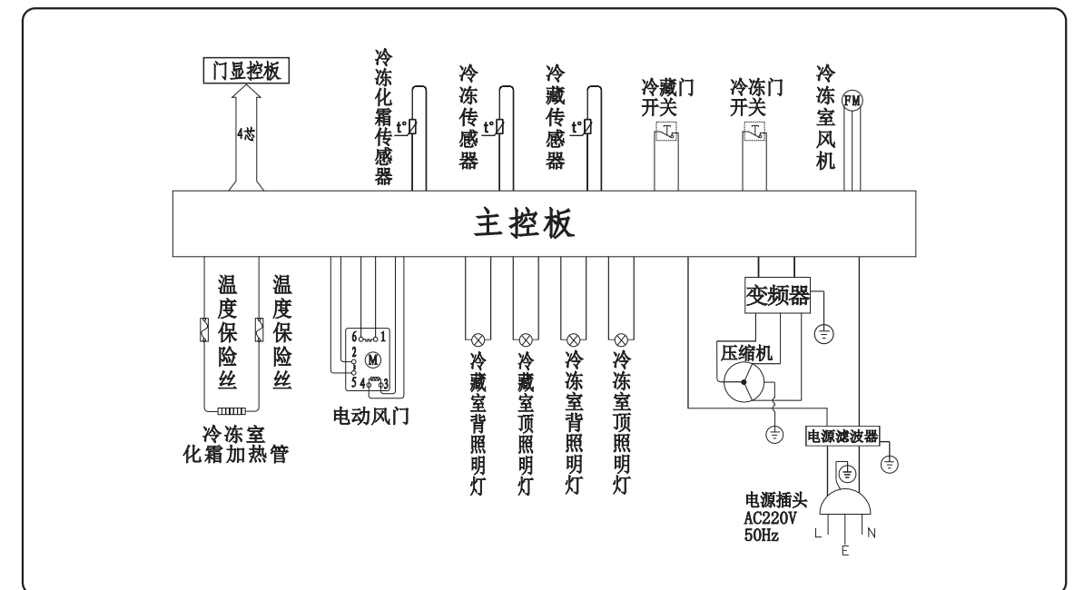
电路图 (BCD-592WDBZW)
